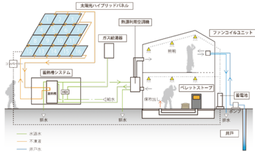
5. O邸オフグリッドハウスのエネルギー循環イメージ図 6.完成イメージ
